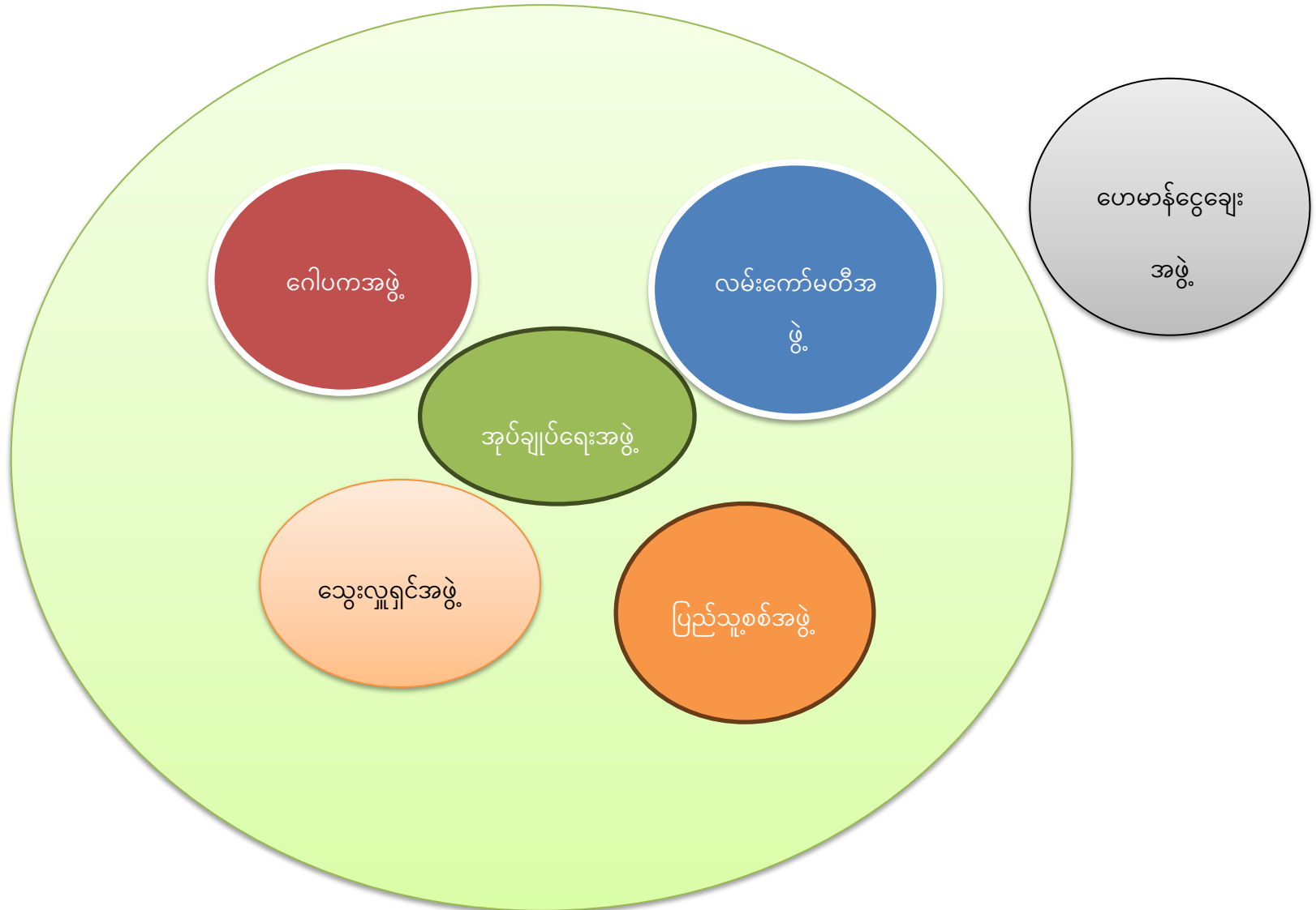
Venn Diagram
